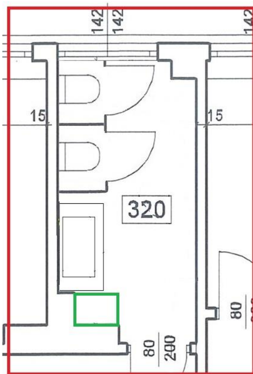
Rysunek 7 Propozycji przebudowy łazienek na III piętrze budynku II US w Toruniu pomieszczenia 320
