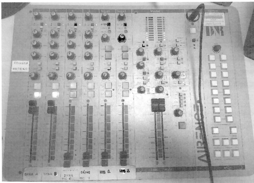
Fot. 1. Widok wycenianej konsoli transmisji radiowej (jednostka główna).
