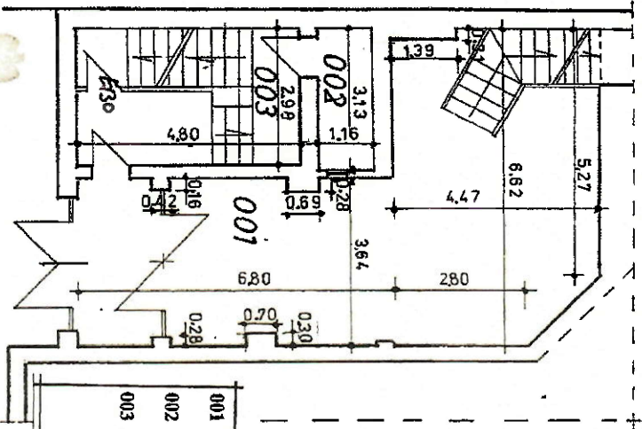
RZUT PARTERU
